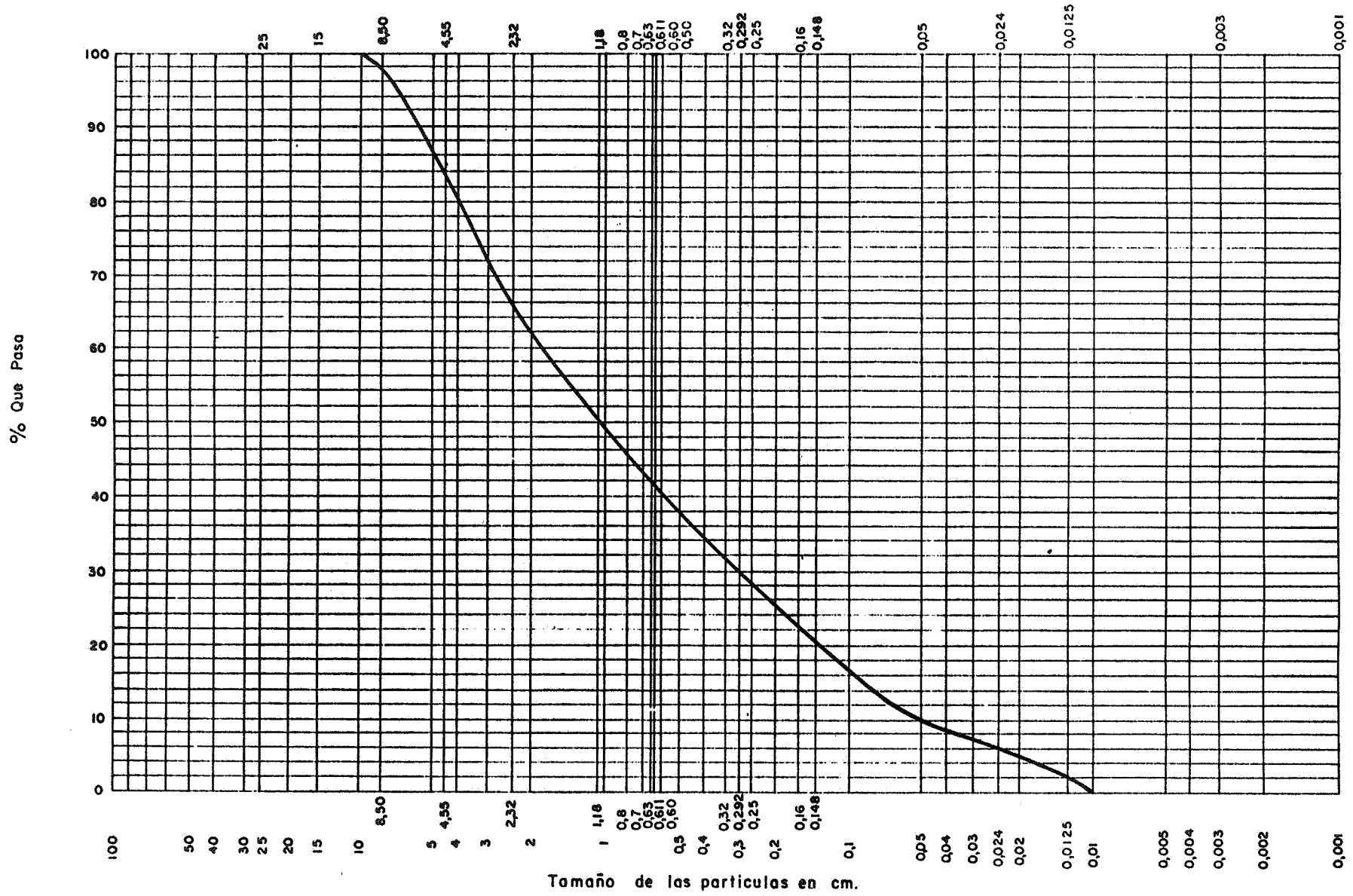
Curva Granulométrica Rio Guadalmedina entre P.K.1800 y P.K.3000
